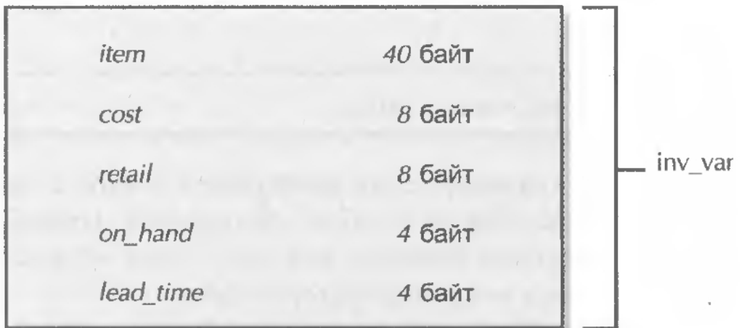
Рис. 10.1. Размещение структурной переменной inv_var в памяти компьютера
