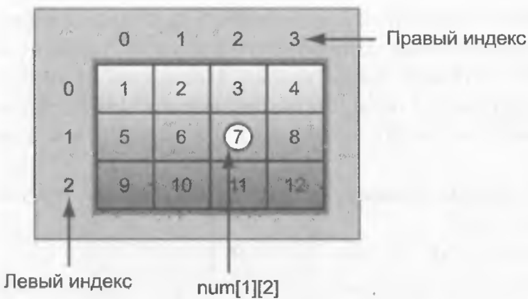
Рис. 5.1. Схематическое представление массива num
