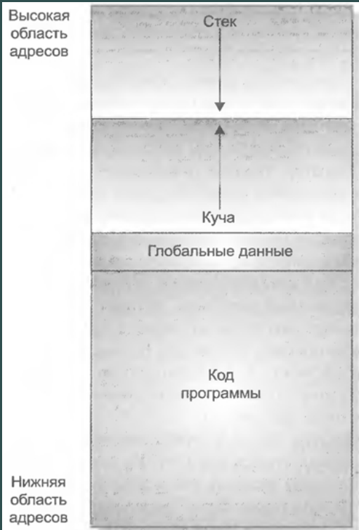
Рис. 9.2. Использование памяти в C++-программе
