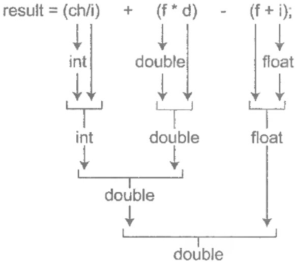
Рис. 3.1. Пример преобразования типов в C++
